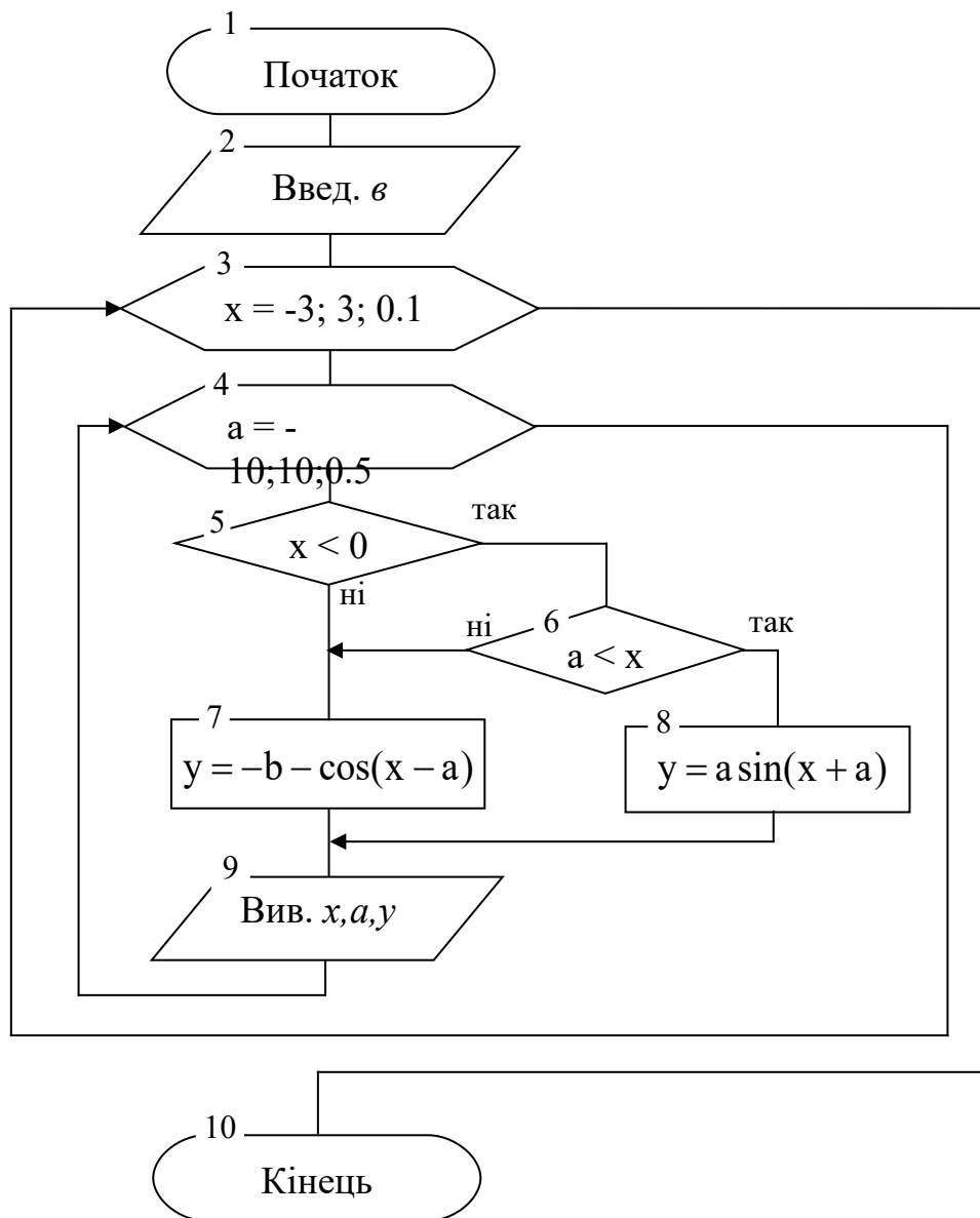
Рисунок 18 – Алгоритм вкладеного циклічного процесу з розгалуженнями
