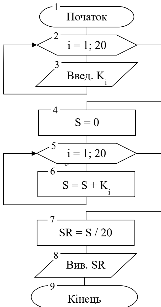
Рисунок 23 – Алгоритм визначення середнього арифметичного значення елементів масиву
