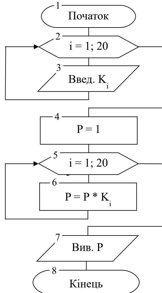
Рисунок 24 – Алгоритм визначення добутку елементів масиву
