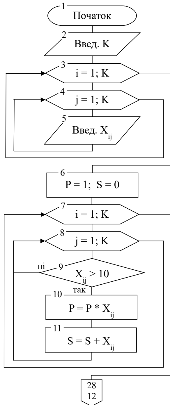
Рисунок 25 – Алгоритм до прикладу 14
