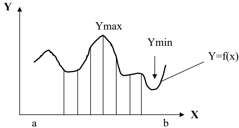
Рисунок 19 – Максимальне та мінімальне значення функції
