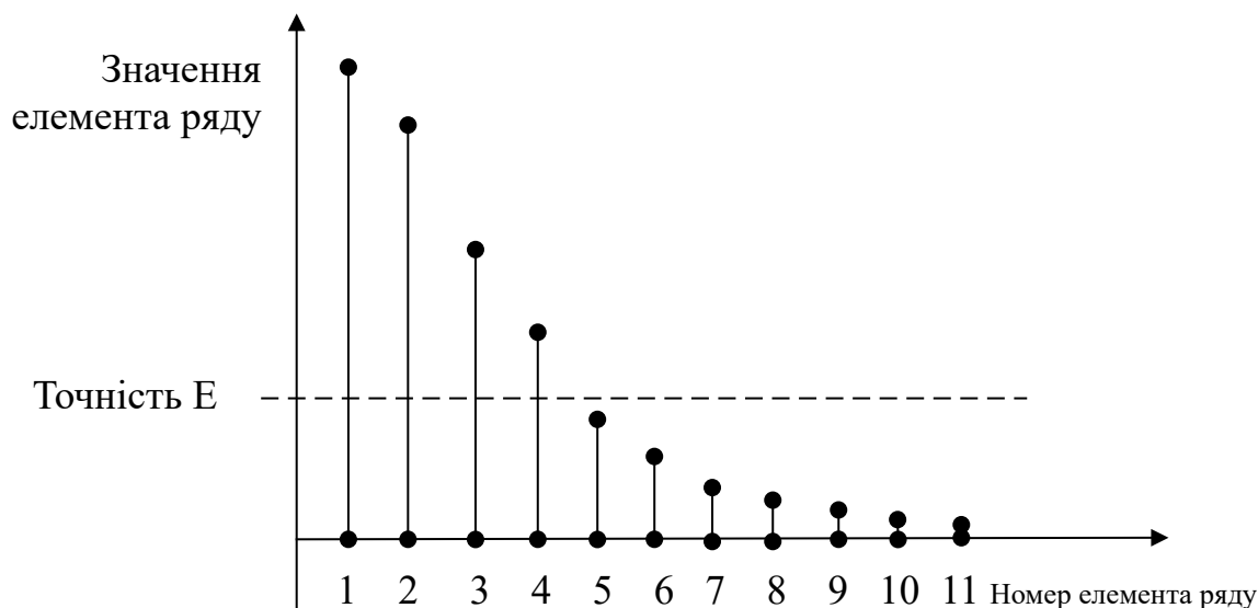
Рисунок 14 – Залежність абсолютного значення елемента ряду, що збігається, від його номера
